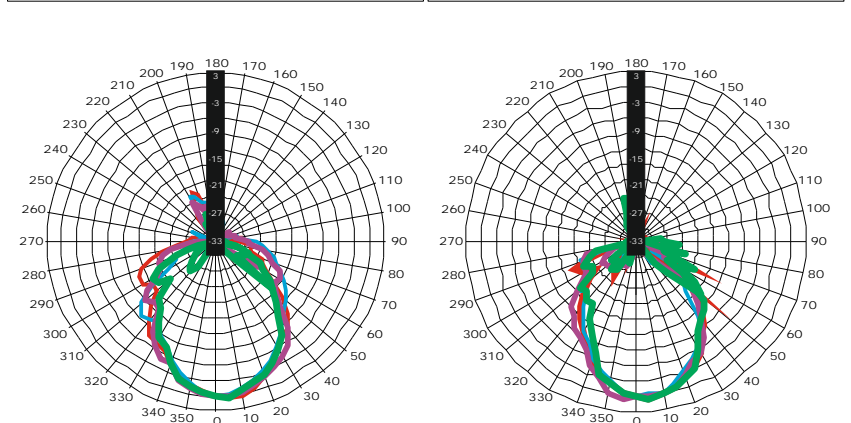
VERTICAL POLAR DIAGRAM Legend: 4000 (cyan), 5000 (red), 6300 (purple), 8000 (green), 9000 (cyan), 10000 (orange), 12500 (magenta), 14000 (dark green)
